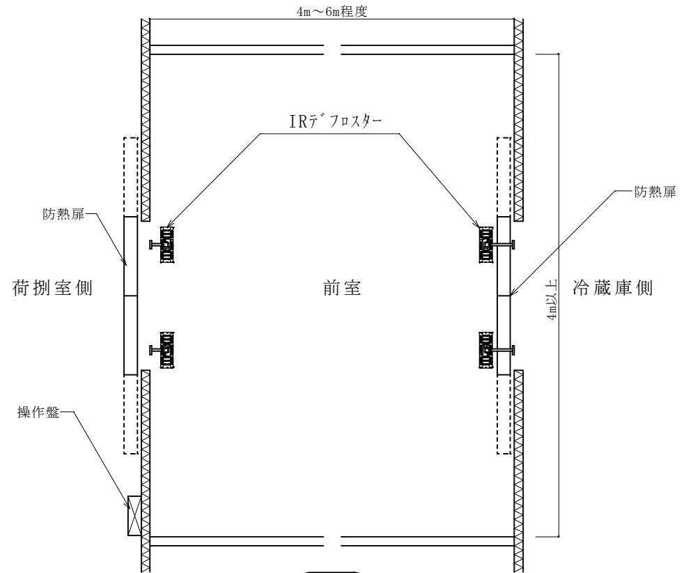
平面図
