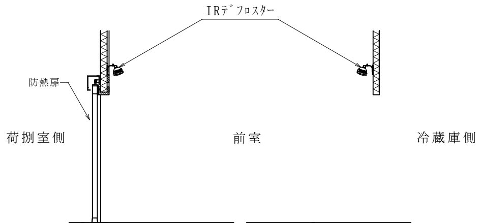
断面図
