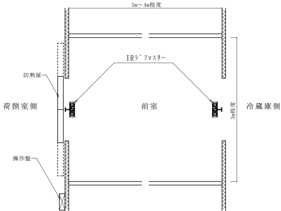
平面図
