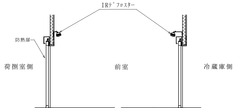
断面図
